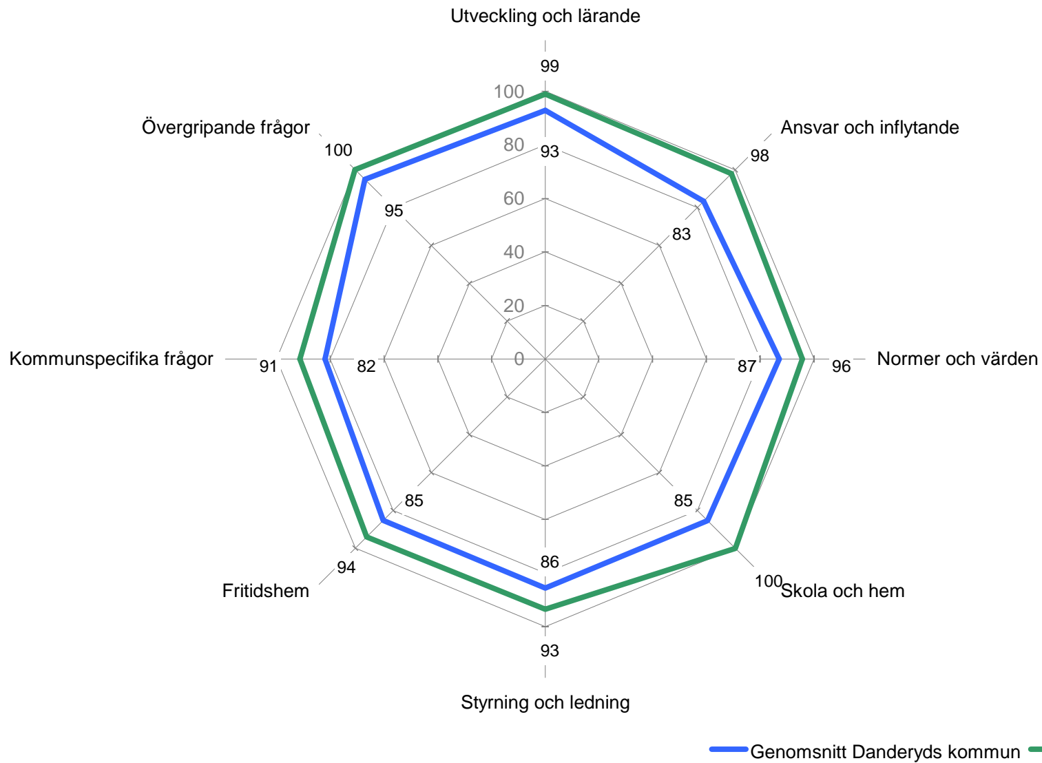
Genomsnittlig andel 'Stämmer bra' per målområde
